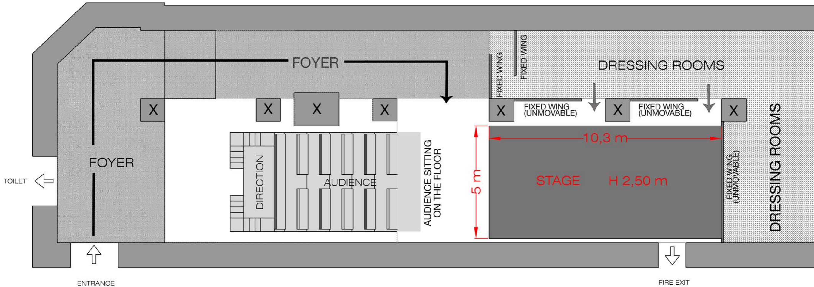
TEATRO DELLE SEI - PLAN 1:100
